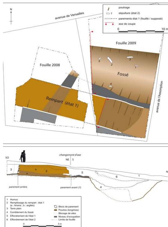
Fig. n°1 : Plan et coupe simplifiés de l'état 1
